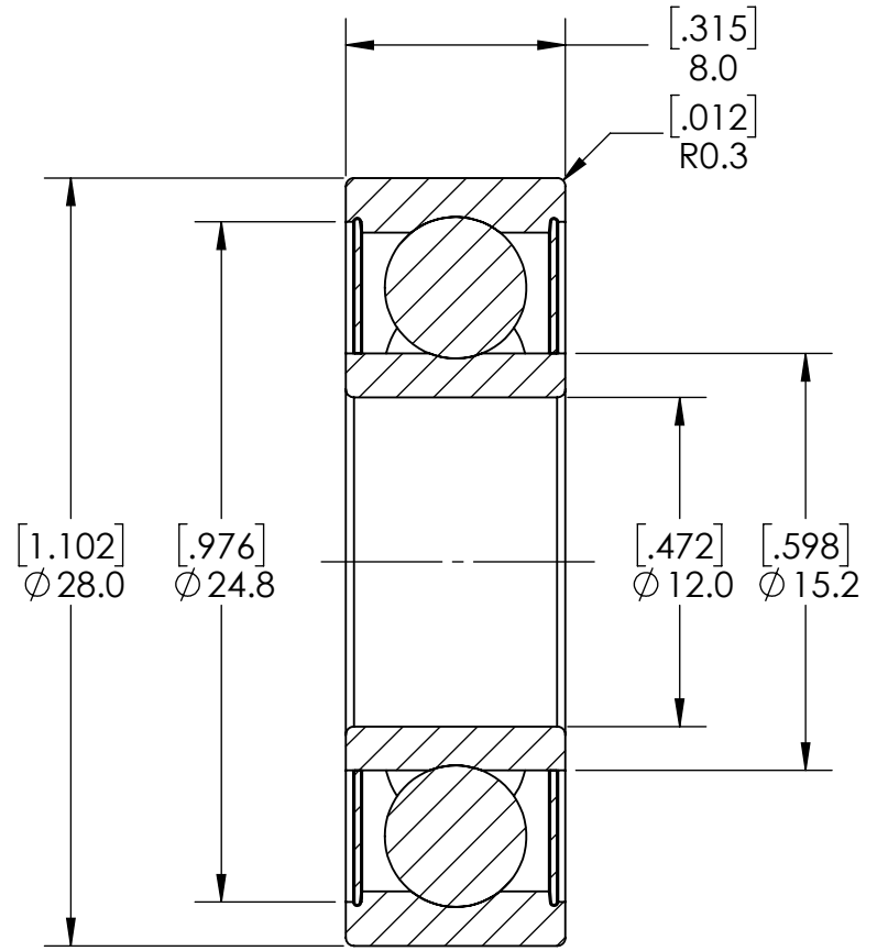
SECTION A-A
